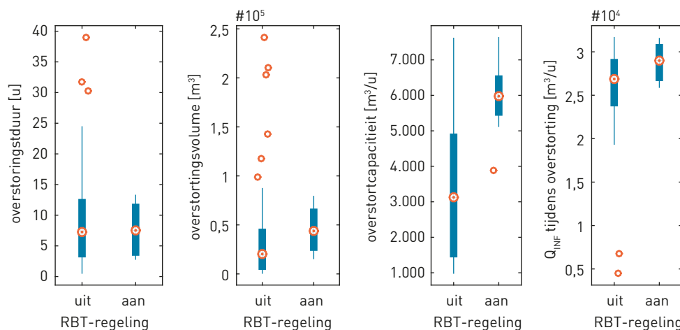
Figuur 4.5 Boxplots voor diverse RBT-beoordelingsparameters voor alle overstortingen
