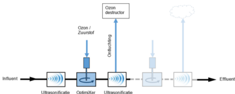
BLOKSCHEMA O_3 + ULTRASOUND
