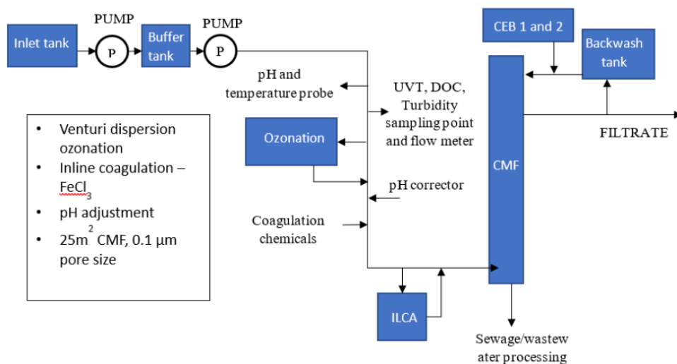
FIGUUR 3.15 BLOKSCHEMA OZON MET KERAMISCHE MICROFILTRATIE
