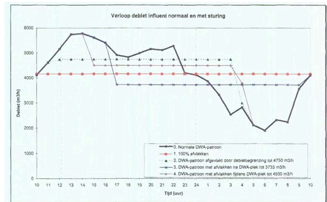
Afbeelding 7 Verloop van debiet door verschillende sturingsstrategieën m.b.t. afvlakking DWA-patroon
