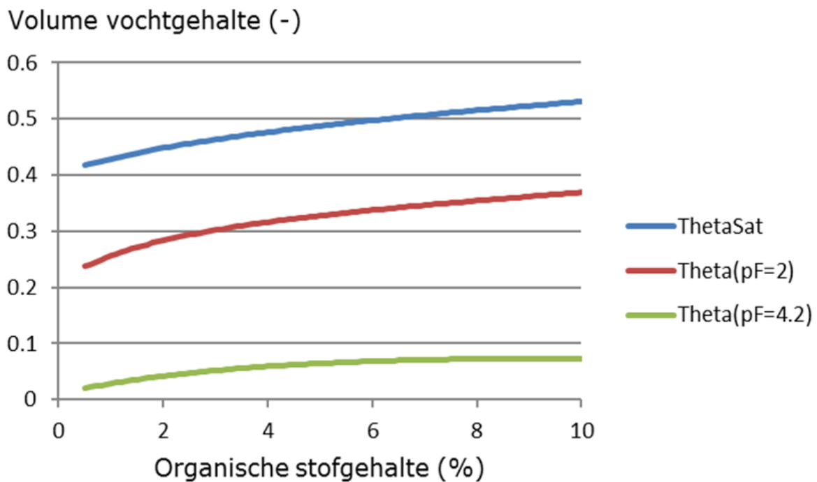
Figuur 4. Verloop van het volume vochtgehalte bij verzadiging, bij pF 2 (veldcapaciteit) en bij pF 4.2 (verwelkingspunt) met het organische stofgehalte.
