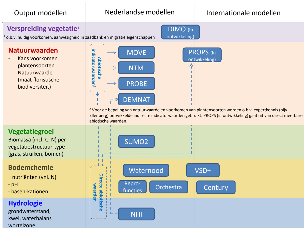
Figuur 6. Overzicht van modelconcepten terrestrische vegetatie bij KWR (PROBE, Waternood, Orchestra, Century), Alterra (DIMO, PROPS, MOVE, NTM, SUMO2, VSD+, NHI) en Deltares (DEMSTAT, NHI).
