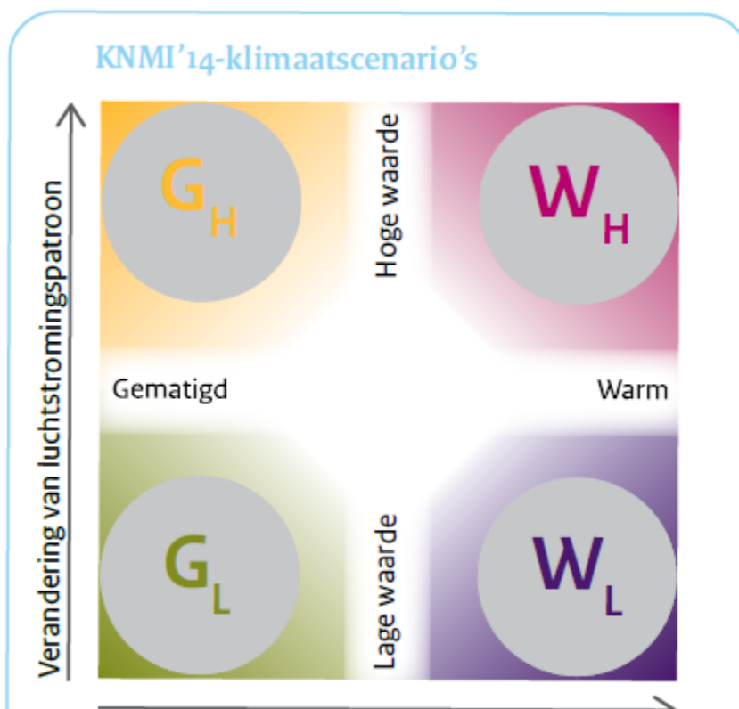
Figuur 2. Overzicht van de vier klimaatscenario's van 2014 van het KNMI (Bron: ( KNMI, 2014 ))
