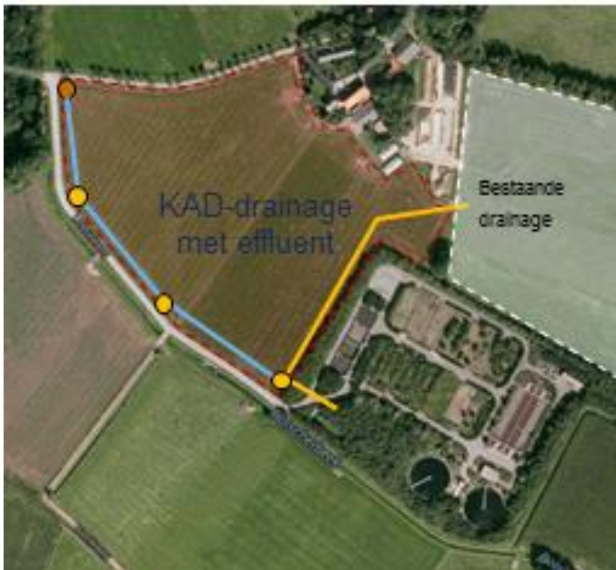
Figuur 3. Proefperceel voor subirrigatie met rwzi-effluent te Haaksbergen.
