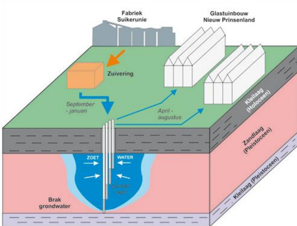
Figuur 5. Vergaande zuivering van Suikerunie effluent tot gietwater en tijdelijke opslag in de ondergrond bij glastuinbouwgebied Nieuw Prinsenland (Zuurbier en Ros 2016).
