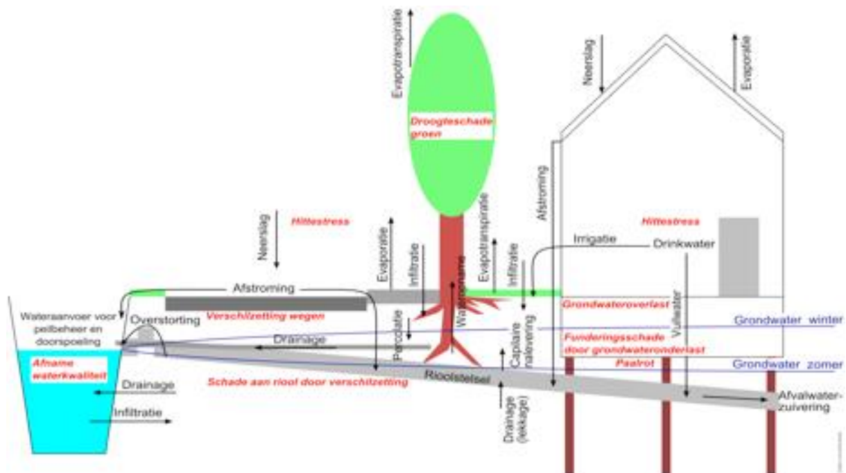
Figuur 3. Watersysteem op straatniveau in laag Nederland
