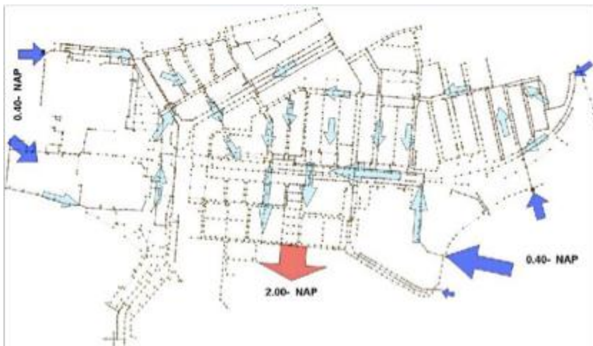
Figuur 5. Watersysteem Amsterdamse Rivierenbuurt ( Jacco Kroon, 2011 )
