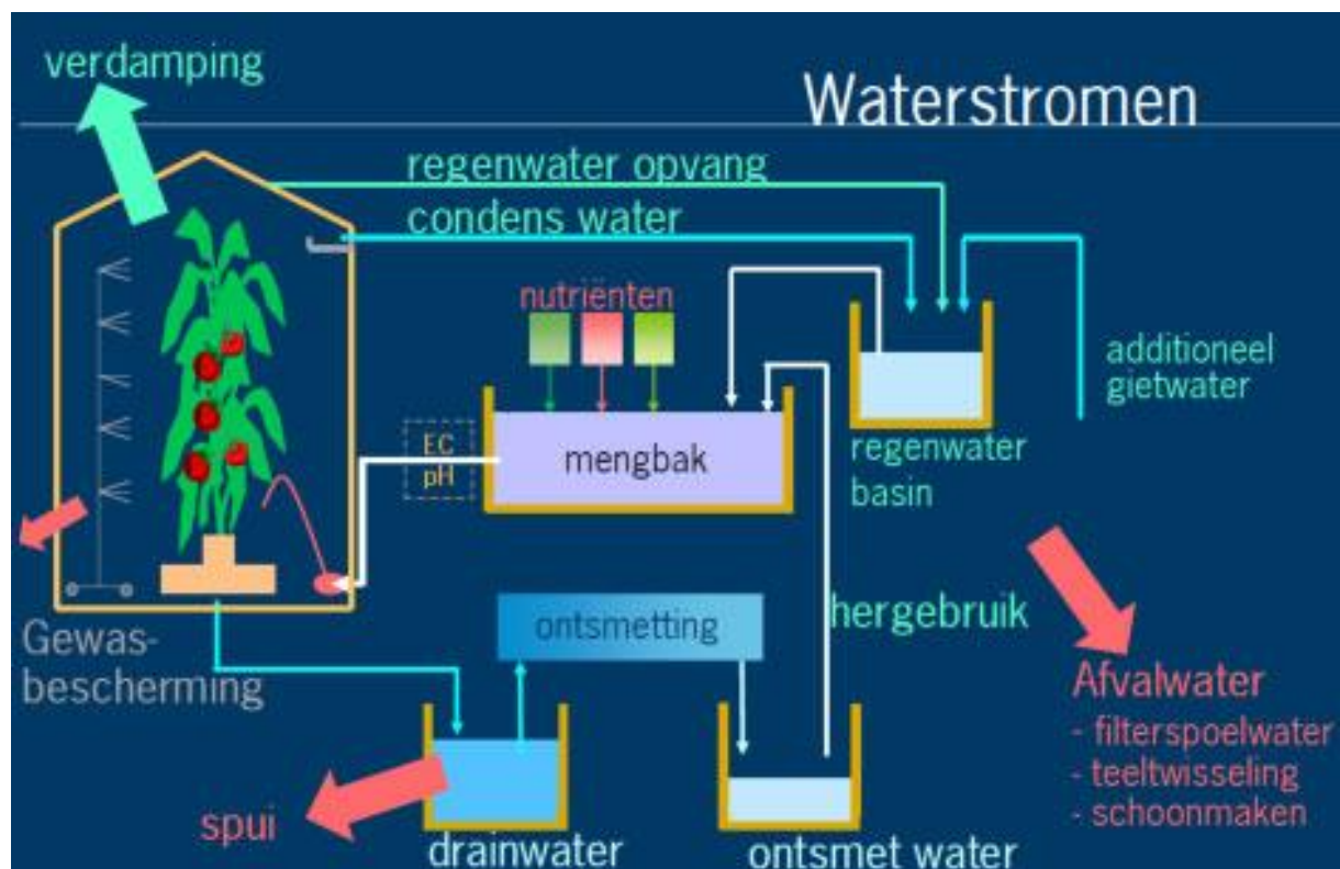
Figuur 2. De waterstromen en de rol van het regenwater bassin in de geavanceerde glastuinbouw (Bron: van Os, 2010)
