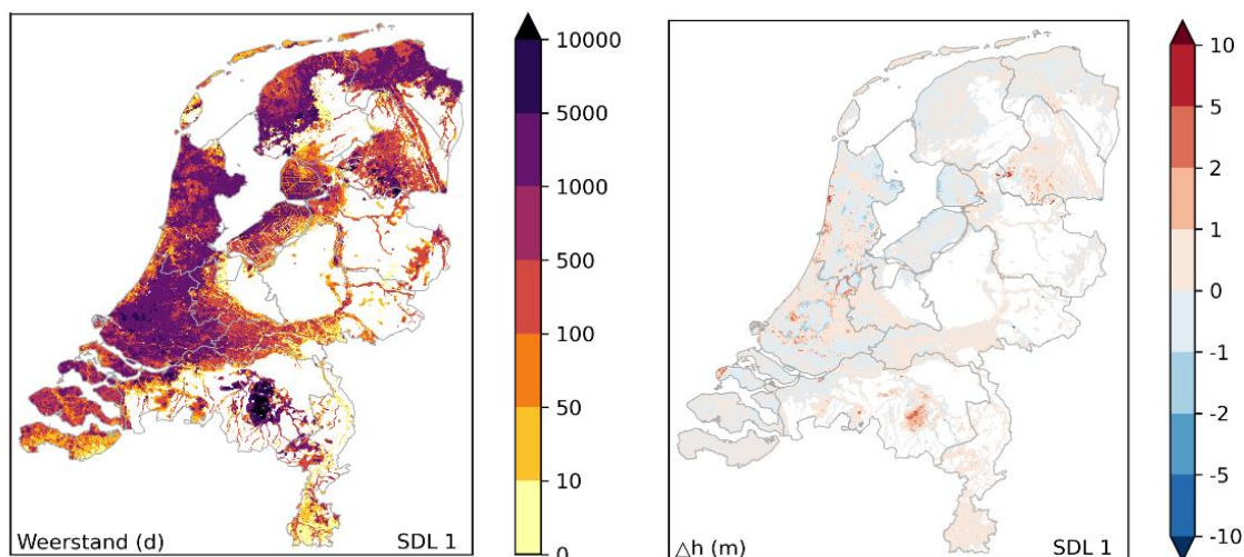
Figuur 5 Links: Illustratie van de weerstand over de eerste scheidende laag (in dagen). Rechts: stijghoogteverschil over de eerste scheidende laag (in meters). Blauw is kwel, rood is infiltratie. Waar SDL1 ontbreekt is de kleur wit. De kaarten voor de overige scheidende lagen en risicokaarten zijn terug te vinden in de geohydrologische beschermkaarten (TNO, 2022). 6
