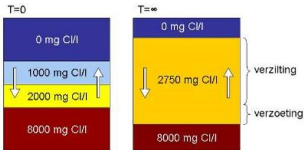
Figuur 6 Illustratie van mogelijke effect vermenging veroorzaakt door een OBES systeem in een watervoerend pakket met een niet lineaire chloride verdeling. Uit: Meer Met Bodemenergie (2012a).
