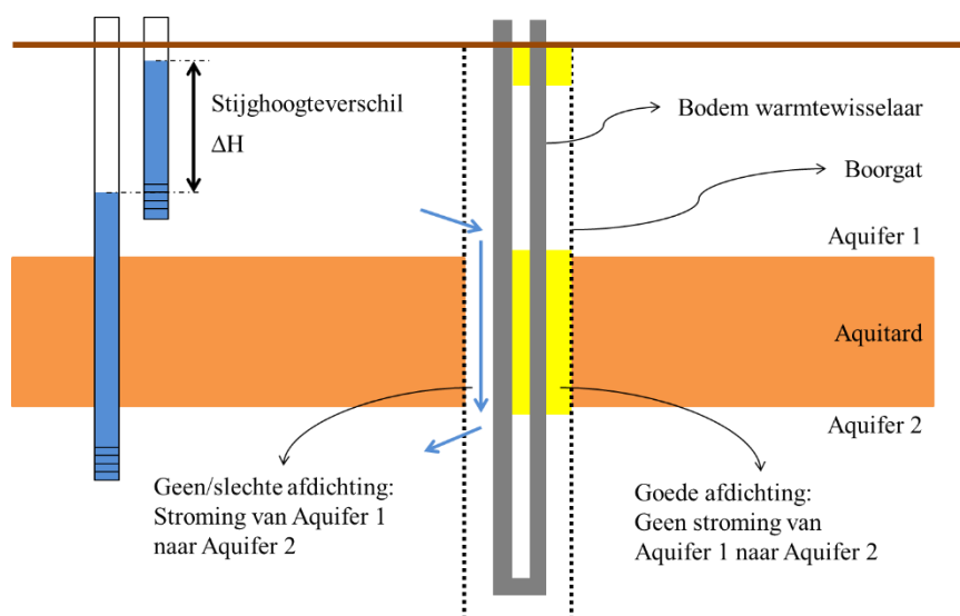
Figuur 4 Schematische weergave van kortsluitstroming in een inadequaat afgedichte boorgat, in dit geval een lus van een GBES.
