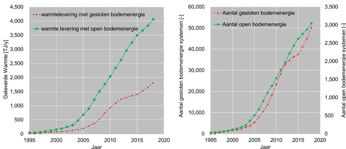
Figuur 1 Links: Totaal geleverde warmte per jaar per type bodemenergiesysteem. Rechts: Ontwikkeling aantal geïnstalleerde bodemenergiesystemen. Bron: Vereniging Warmtepompen en CBS. https://www.duurzaamverwarmd.nl/trendrapport/ . NB. Bij open bodemenergiesystemen zitten er vaak meerdere warmtepompen aan 1 systeem, uit het Landelijk Grondwater Register weten we dat er circa 3000 open systemen zijn.
