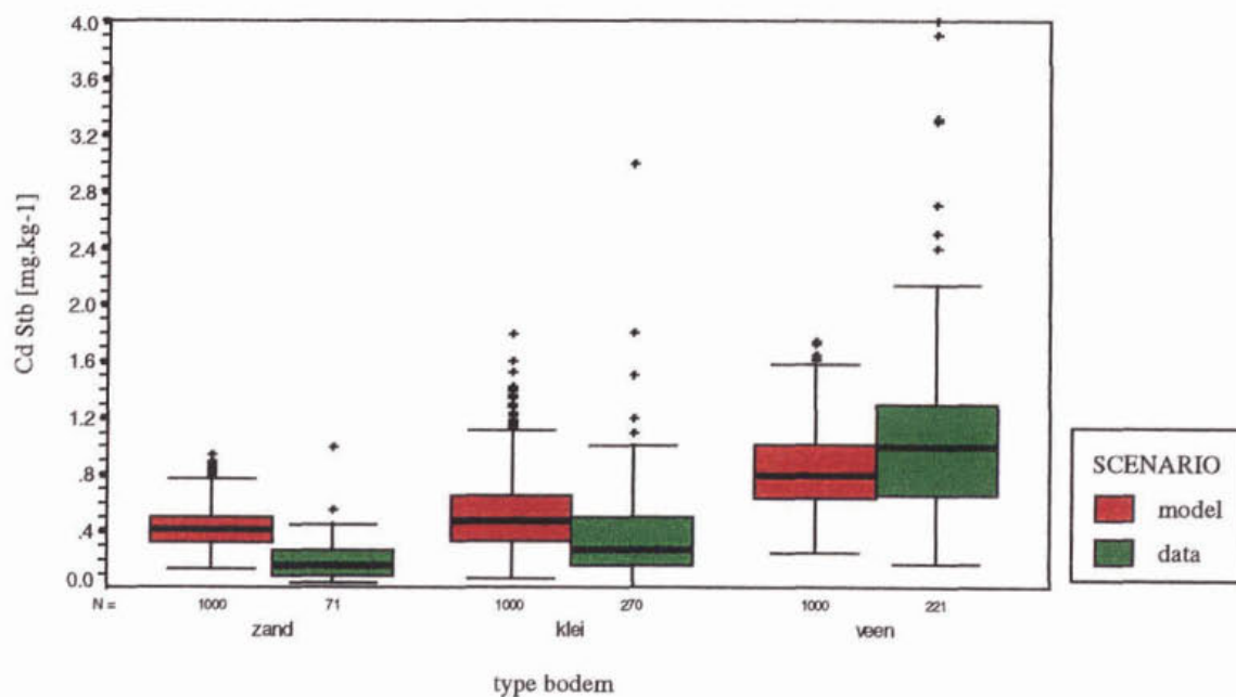
Figuur 5.3 Vergelijking van berekende en gemeten gehalten cadmium omgerekend naar standaardbodem in zand-, klei- en veensloten
