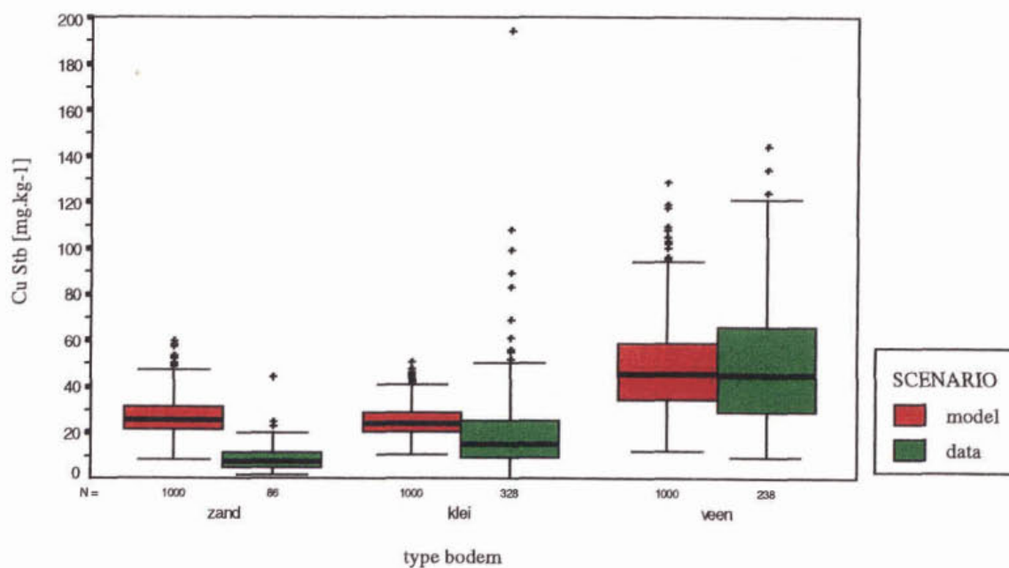
Figuur 5.4 Vergelijking van berekende en gemeten gehalten koper omgerekend naar standaardbodem in zand-, klei- en veensloten
