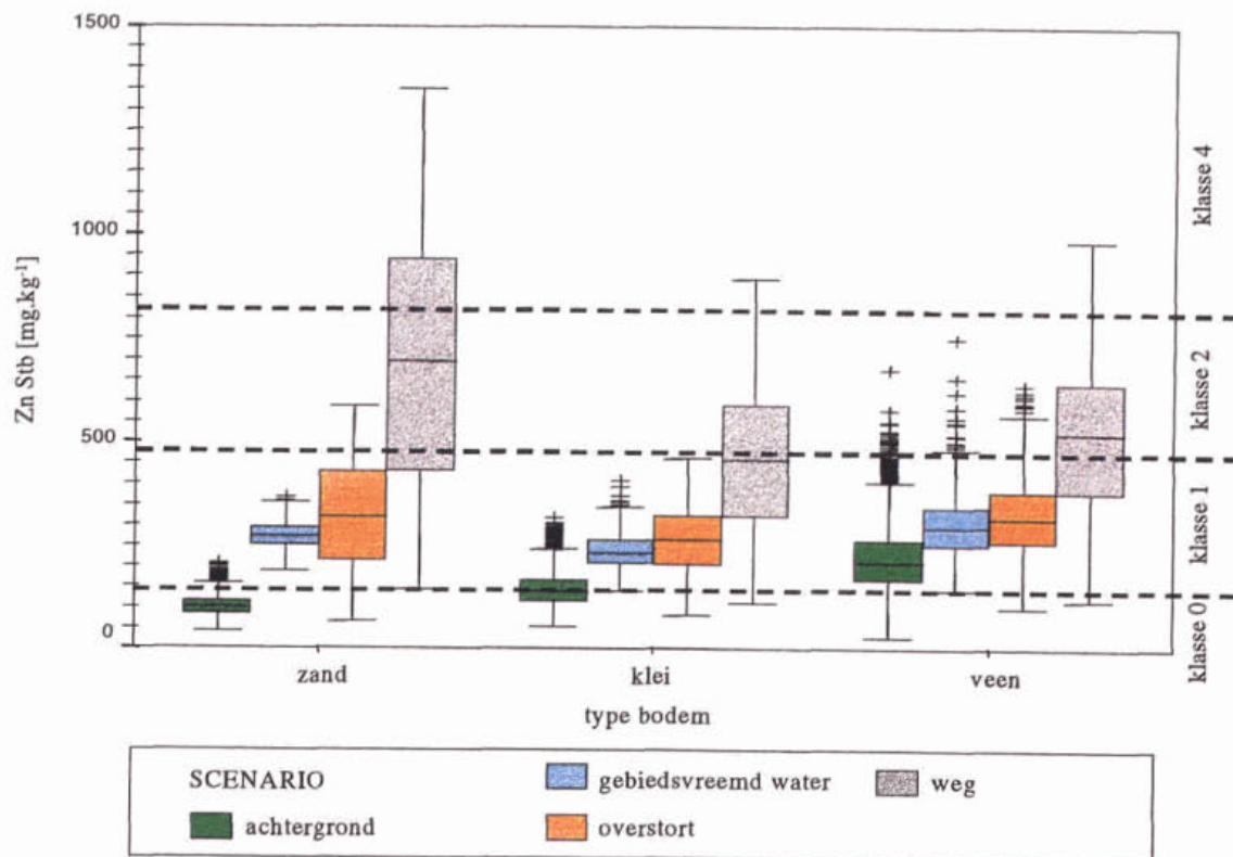
Figuur 6.12 Gehalten zink omgerekend naar standaardbodem in zand-, klei- en veensloten bij verschillende typen hoge belasting.
