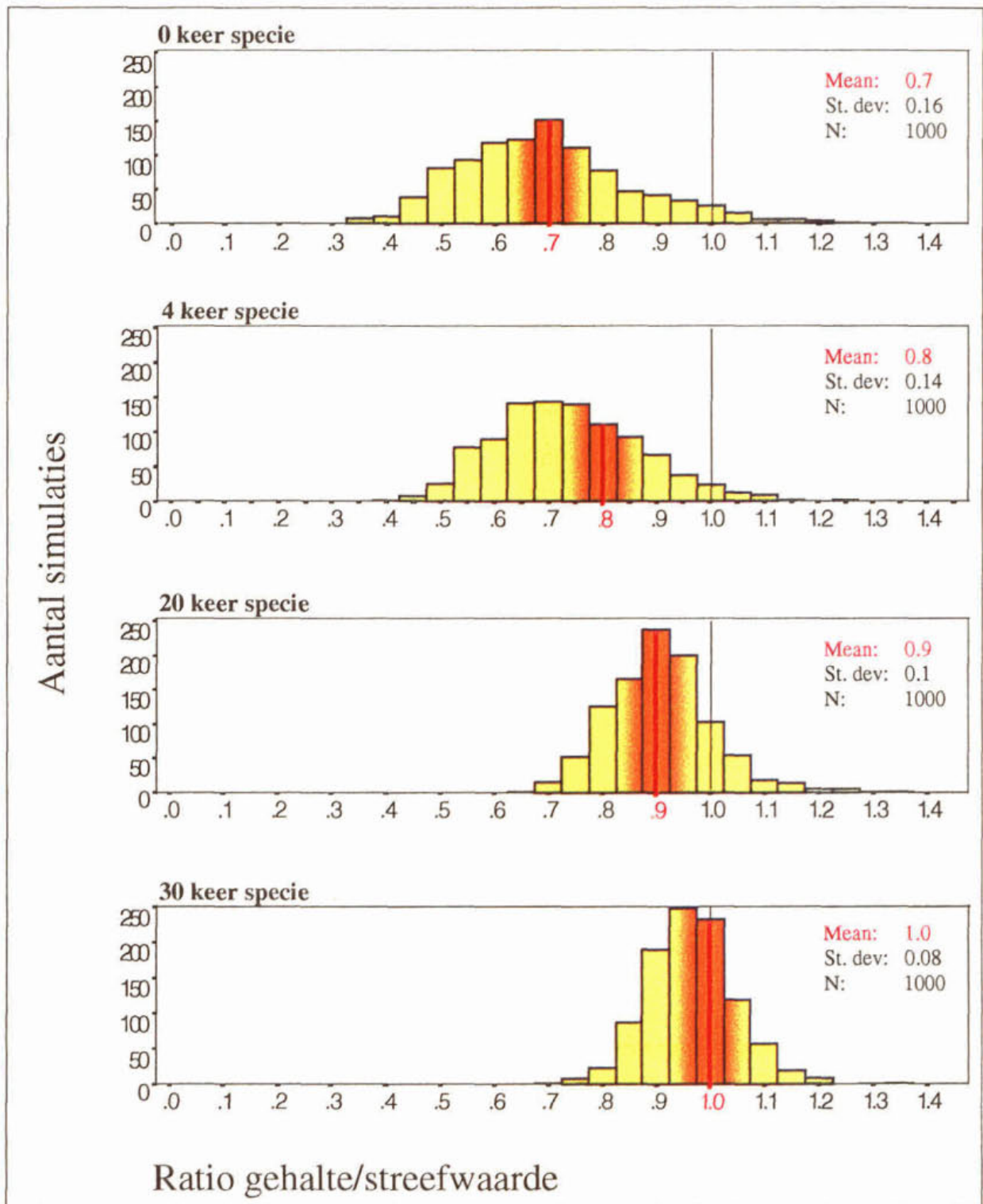
Figuur 5.5. Ontwikkeling metaalgehalte in landbodern na 0, 4, 20 en 30 keer opbrengen bovengrens klasse 0 specie met betrekking tot zink ( 140 \text{ mg}\cdot\text{kg}\cdot\text{ds}^{-1} standaard bodern) op bouwland op klei.
