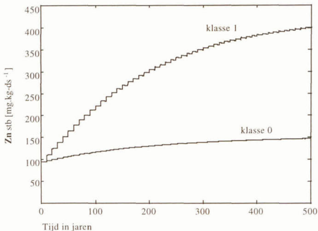
Figuur 4.2. Verloop gehalte Zn in landbodem (bouwland op klei) na opbrengen van klasse 0 en 1 specie gedurende 500 jaar. Kwaliteit specie (stb) [ \text{mg Zn} \cdot \text{kg-ds}^{-1} ]: klasse 0 = 140; klasse 1 = 480.
