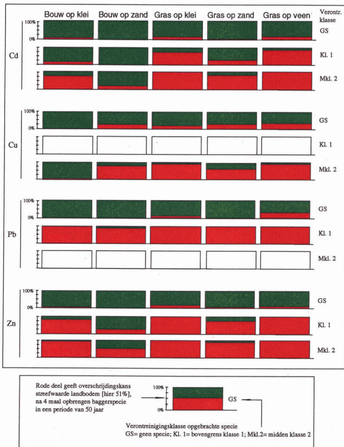
Figuur C1. Kans op overschrijding van de streefwaarde [0-100%] zonder het opbrengen van specie en na 4 maal opbrengen van klasse 1 of "midden klasse 2" specie binnen een periode van 50 jaar.
