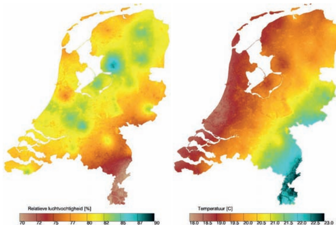
FIGUUR 11 RELATIEVE LUCHTVOCHTIGHEID (LINKS) EN TEMPERAATUUR (RECHTS) VLAKDEKKEND VOOR HEEL NEDERLAND BEREKEND M.B.V. METEOLOOK. VOORBEELD VOOR 22 JULI 2009. (BRON: WATERWATCH)
