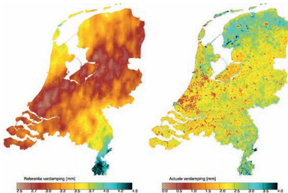
FIGUUR 6 REFERENTIEVERDAMPING VOLGENS PENMAN-MONTEITH (LINKS) EN ACTUELE VERDAMPING VOLGENS SEBAL (RECHTS) ZOALS DEZE WORDEN BEREKEND DOOR WATERWATCH. VOORBEELD VOOR 22 JULI 2009. N.B. DE KLEURENSCHAAL VERSCHILT PER PLAATJE
