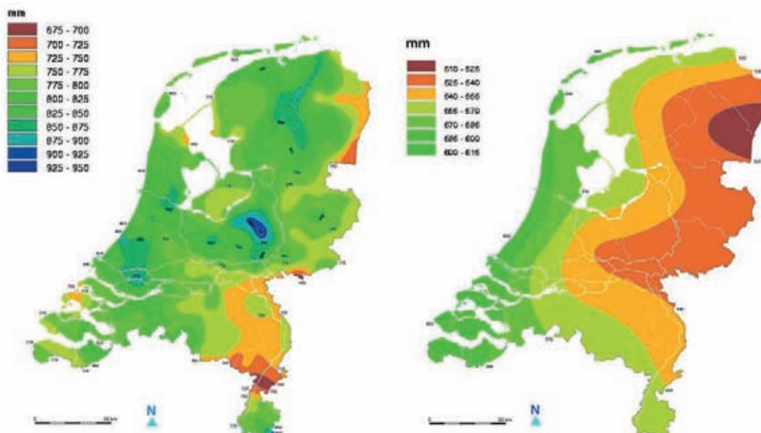
FIGUUR 1 LANGJARIG GEMIDDELTE JAARLIJKSE NEERSLAG (LINKS) EN REFERENTIEVERDAMPING VOLGENS MAKKINK (RECHTS). (BRON: KNMI, 2000)
