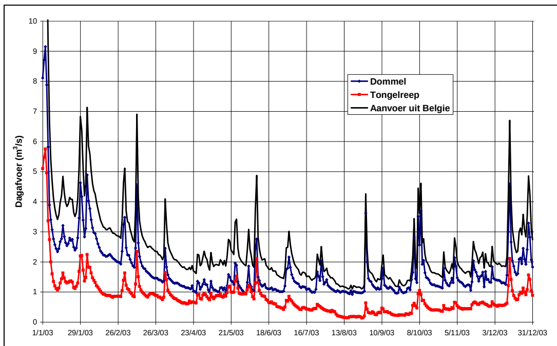
Figuur 3.3 Afvoer van Dommel en Tongelreep bij de Belgische grens
