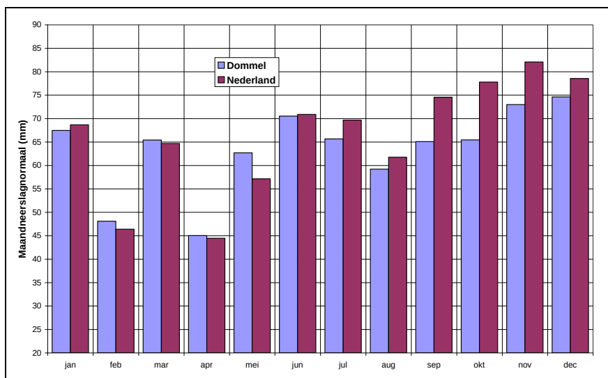
Figuur 2.2 Maandneerslagnormalen voor beheergebied van waterschap de Dommel en Nederland
