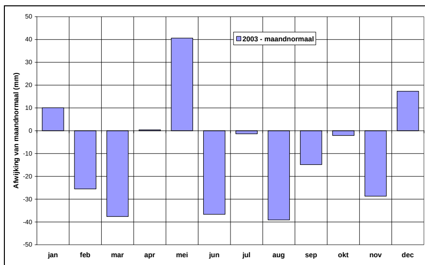
Figuur 2.4 Afwijking van de maandneerslagsommen van 2003 van de maandnormalen
