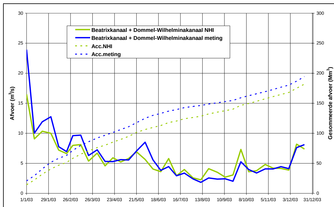
Figuur 3.13 Gemeten en berekende som van de afvoeren van Beatrixkanaal en Dommel-Wilhelminakanaal, 2003
