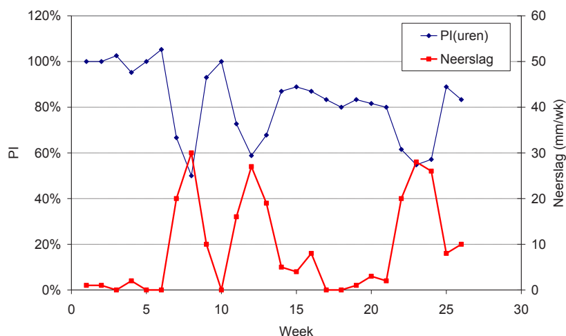
FIGUUR 5.2 VOORBEELD DATA VAN EEN PI O.B.V. DRAAIUREN EN DE GEMETEN NEERSLAG
