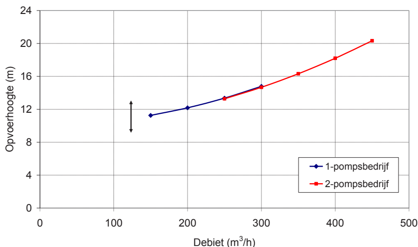
FIGUUR 5.1 SYSTEEMKARAKTERISTIEK EN HET EFFECT VAN DE STATISCHE OPVOERHOOGTE (ZWARTE PIJL)
