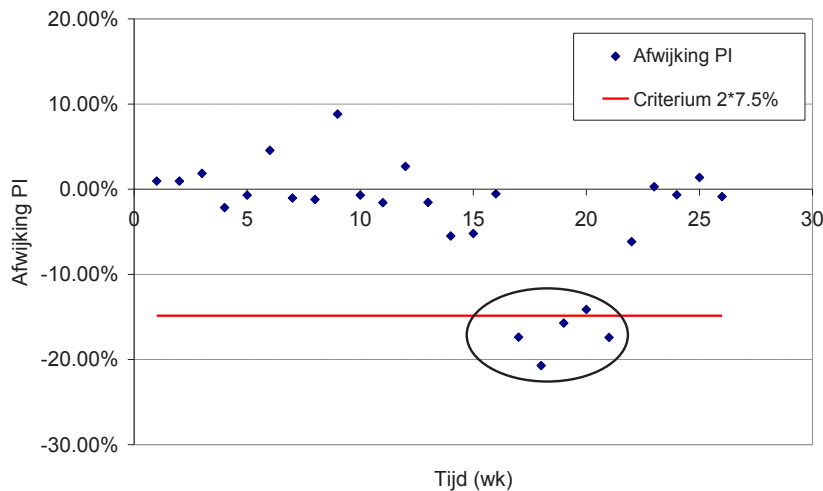
FIGUUR 5.4 AFWIJKING VAN DE PI T.O.V. DE VERWACHTE CORRELATIE TUSSEN NEERSLAG EN PI
