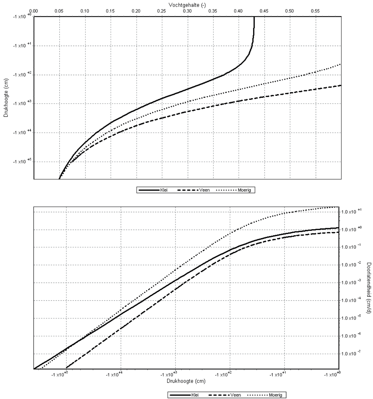
FIGUUR 10 DE WATERRETENTIEKARAKTERISTIEK (A) EN HYDRAULISCH GELEIDINGSVERMOGEN (B) VAN DE GEBRUIKTE BODEMMATERIALEN.
