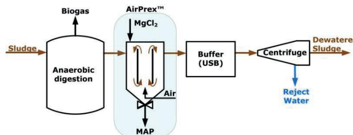
BLOKSCHEMA SLIBGISTINGSINSTALLATIE EN STRUVIETREACTOR RWZI AMSTERDAM WEST
