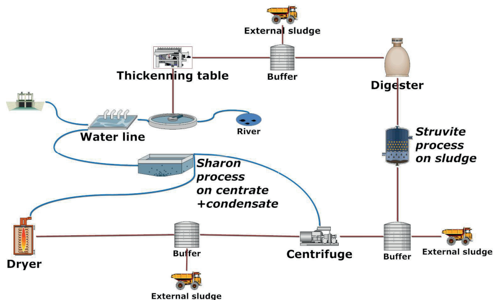
SCHEMA RWZI LEUVEN
