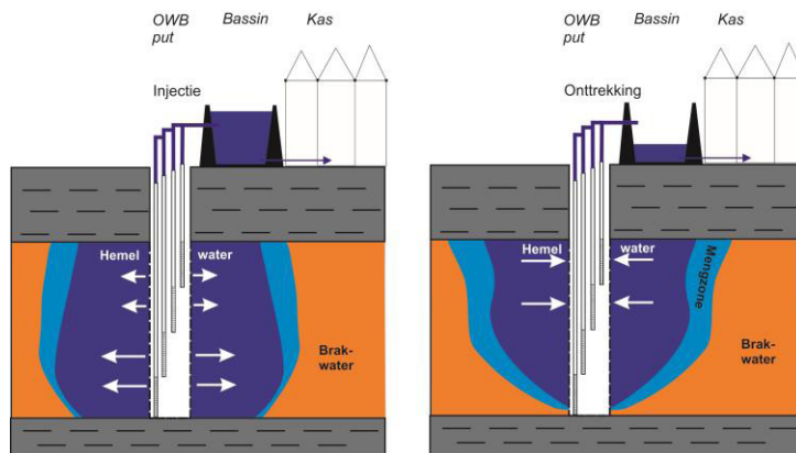
FIGUUR 10 TOEPASSING VAN DE FRESHMAKER VOOR ONDERGRONDSE WATERBERGING. MET HORIZONTALE PUTTEN WORDT ZOWEL ZOETWATER GEÏNJECTEERD EN ONTTROKKEN, ALSMEDE DIEPER ZOUTWATER AFGEVANGEN. HET ZOETE WATER KOMT THANS VANUIT HET OPPERVLAKTewater (NA ZANDFILTRATIE), HET ZOETE WATER WORDT GELOOSD OP HET OPPERVLAKTewater.
