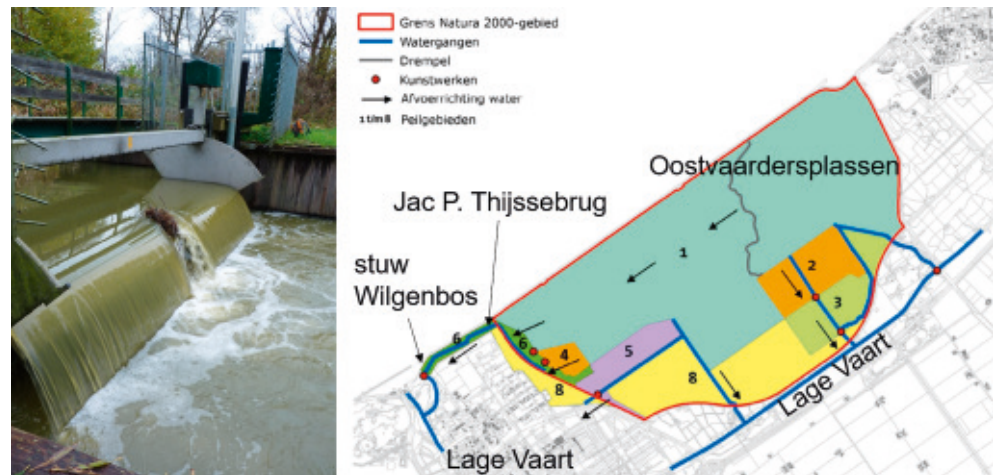
Figuur 9.1 Overzicht afwatering Oostvaardersplassen (rechts) en stuw Wilgenbos (links)
