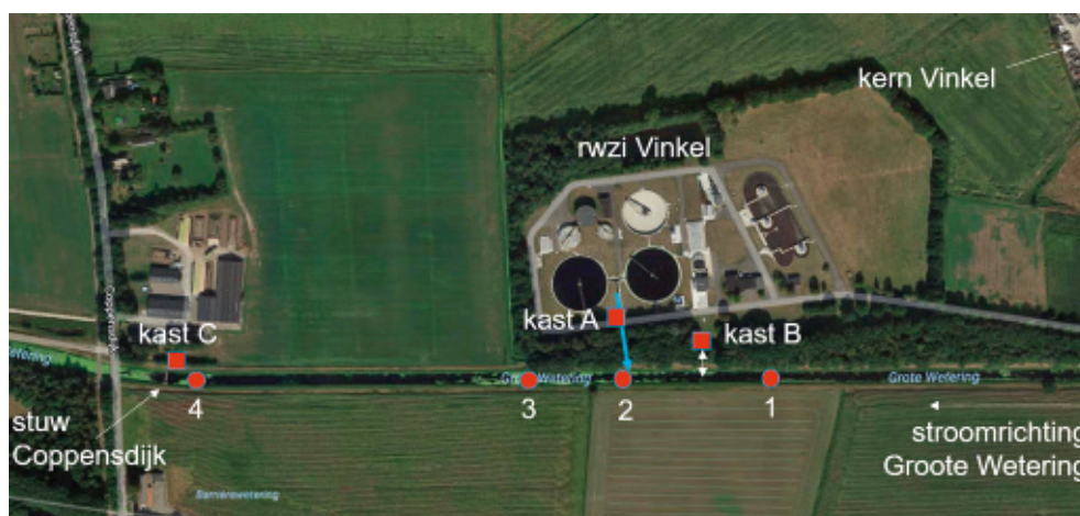
Figuur 4.1 Topografisch overzicht rondom rwzi Vinkel met lozingslocatie in Groote Wetering en benedenstroomse stuw
