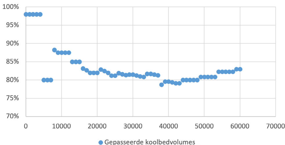
FIGUUR 5.3 GEPASSEERDE KOOLBEDVOLUMES NA START FILTER 1 EN HET TOTALE VERWIJDERINGSRENDEMENT VAN ALLE FILTERS IN BEDRIJF IN KOOLBEDVOLUMES GEPASSEERD NA START FILTER 1
