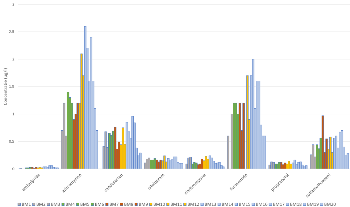
FIGUUR 3.8 KANDIDAAT GIDSSTOFFEN CONCENTRATIE ( \mu\text{g/L} ) IN INFLUENT PILOT (EBCT 15 MIN = GRIJS, EBCT 30 MIN = GROEN, EBCT 20 MIN = ROOD, EBCT 17 MIN = GEEL EN EBCT 23 MIN = BLAUW)
