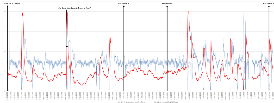
FIGUUR 0.39 TIJDLIJN VAN DRIE BEMONSTERINGEN (BM4, BM5 EN BM6). RODE LIJN IS DE AMMONIUMCONCENTRATIE (MG/L) IN HET INFLUENT VAN DE BODAC FILTER. BLAUWE LIJN IS DE ZUURSTOFCONCENTRATIE (MG/L) IN HET FILTRAAT VAN DE BODAC FILTER
