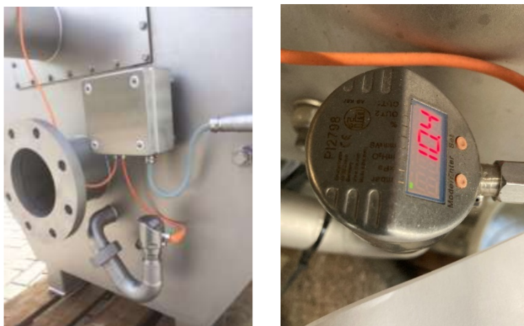
NIVEAUBEWAKING TROMMELZEEF MET DRUKSENSOR
