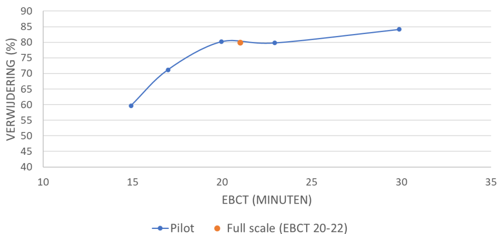
FIGUUR 3.22 GEMIDDELDE VERWIJDERINGSRENDEMENT VAN DE FULL SCALE EN BODAC-OUDE, IN HET GEVAL VAN DE PILOT BIJ VERSCHILLENDE EBCT
