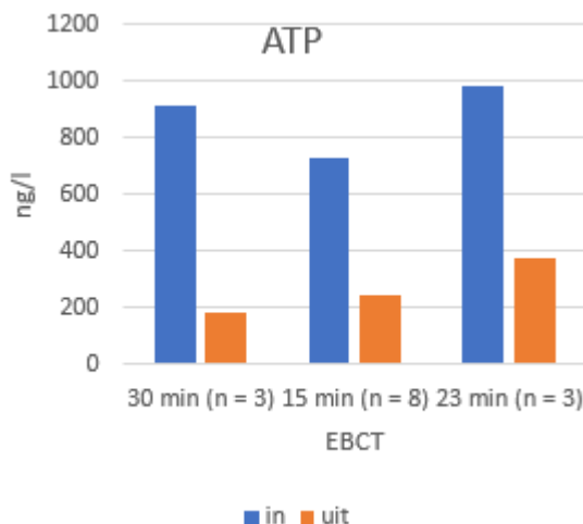
FIGUUR 3.16 GEMIDDELTE ATP CONCENTRATIES IN- EN EFFLUENT
