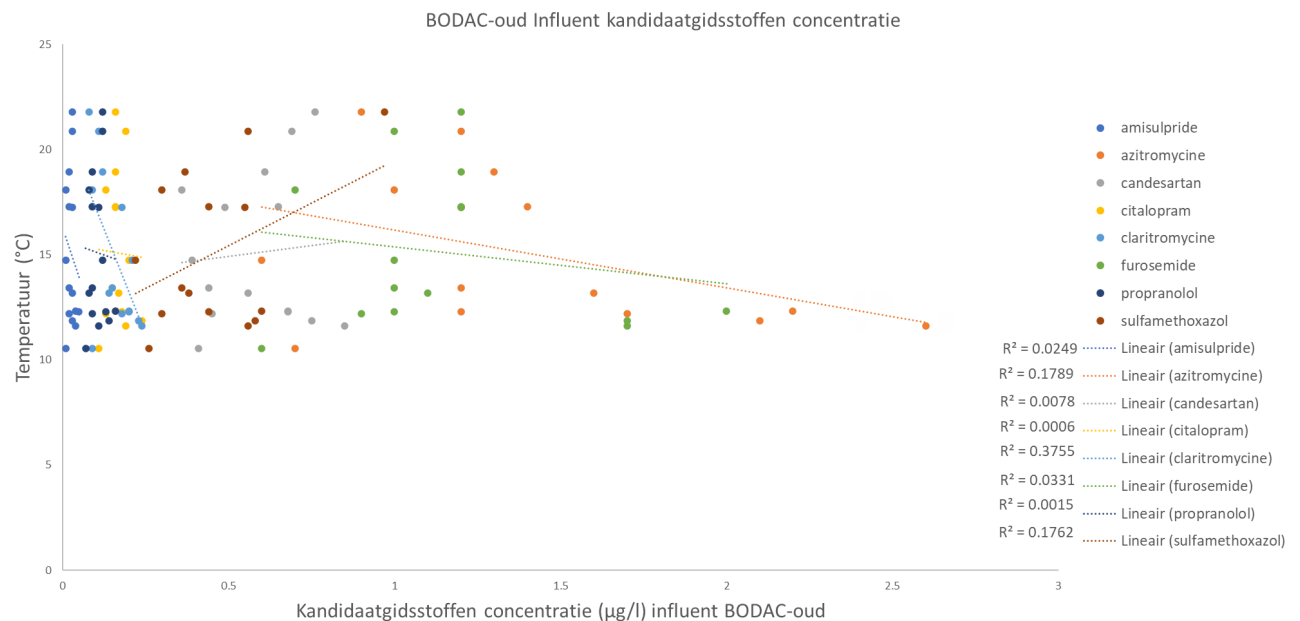
FIGUUR 0.2 CONCENTRATIE KANDIDAATGIDSSTOFFEN ( \mu\text{G/L} ) IN BODAC-INFLUENT UITGEZET TEGEN VOEDINGSWATERTEMPERATUUR ( ^{\circ}\text{C} )
