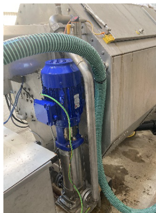
FIGUUR 0.52 SPROEIPOMP
