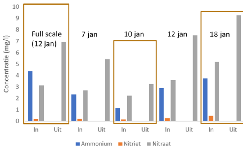
FIGUUR 3.1 NITRIFICATIE RESULTATEN IN DE FULL SCALE INSTALLATIE EN PILOT BODAC-oud TIJDENS DE OPSTARTFASE. IN BEIDE INSTALLATIES KOMT STIKSTOF BINNEN IN DE VORM VAN AMMONIUM, NITRIET EN NITRAAT EN VERLAAT STIKSTOF HET SYSTEEM IN DE VORM VAN NITRAAT
