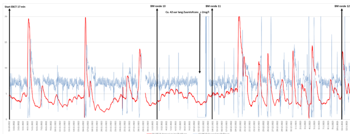
FIGUUR 0.29 TIJDLIJN VAN DRIE BEMONSTERINGEN (BM10, BM11 EN BM12). RODE LIJN IS DE AMMONIUMCONCENTRATIE (MG/L) IN HET INFLUENT VAN DE BODAC FILTER. BLAUWE LIJN IS DE ZUURSTOFCONCENTRATIE (MG/L) IN HET FILTRAAT VAN DE BODAC FILTER
