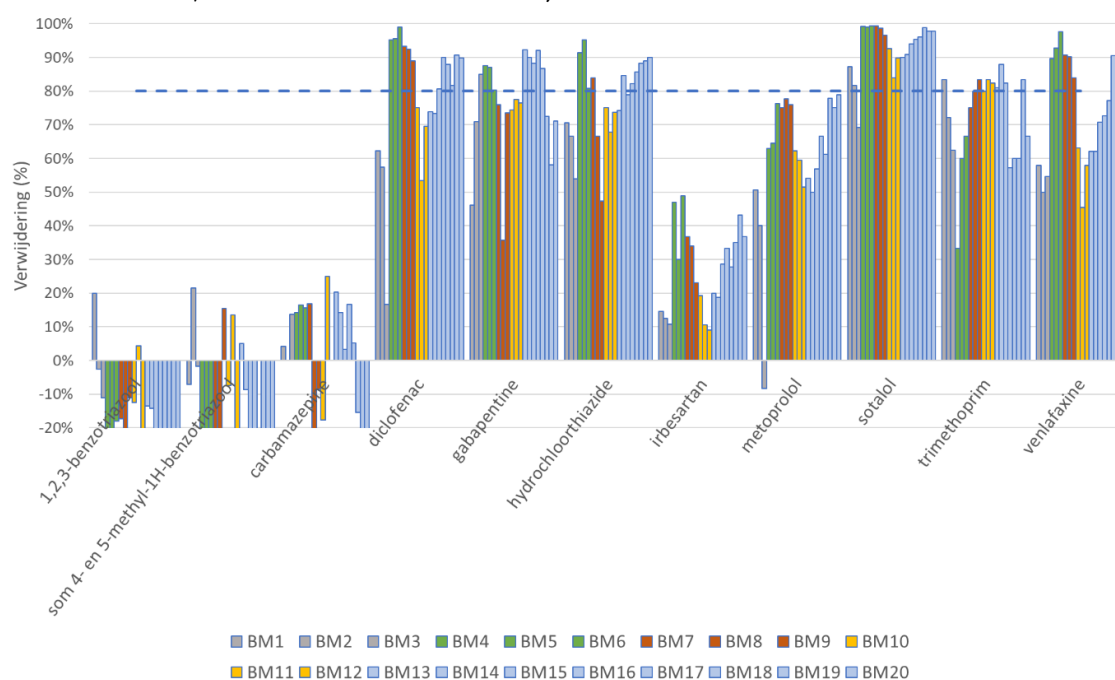
FIGUUR 3.5 GIDSSTOFFEN VERWIJDERINGSRENDAMENT T.O.V. RWZI EFFLUENT (EBCT 15 MIN = GRIJS, EBCT 30 MIN = GROEN, EBCT 20 MIN = ROOD, EBCT 17 MIN = GEEL EN EBCT 23 MIN = BLAUW)
