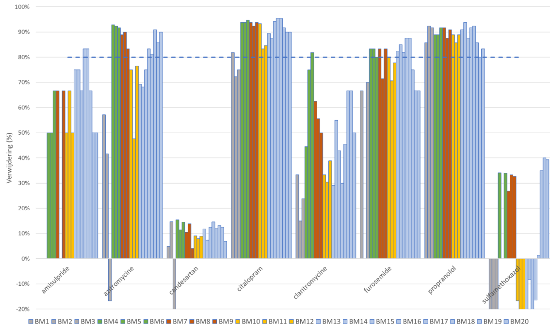
FIGUUR 3.7 KANDIDAAT GIDSSTOFFEN VERWIJDERINGSRENDEMENT T.O.V. RWZI EFFLUENT (EBCT 15 MIN = GRIJS, EBCT 30 MIN = GROEN, EBCT 20 MIN = ROOD, EBCT 17 MIN = GEEL EN EBCT 23 MIN = BLAUW)
