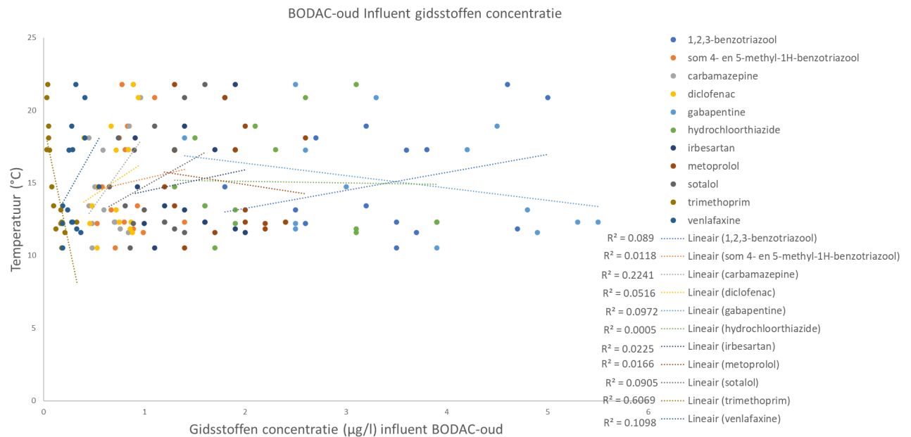
FIGUUR 0.1 CONCENTRATIE GIDSSTOFFEN ( \mu\text{G/L} ) IN BODAC-INFLUENT UITGEZET TEGEN VOEDINGSWATERTEMPERATUUR ( ^{\circ}\text{C} )
