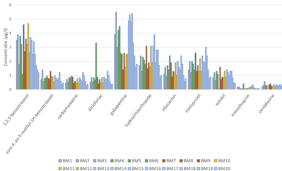
FIGUUR 3.6 GIDSSTOFFEN CONCENTRATIE ( \mu\text{g/L} ) IN INFLUENT PILOT (EBCT 15 MIN = GRIJS, EBCT 30 MIN = GROEN, EBCT 20 MIN = ROOD, EBCT 17 MIN = GEEL EN EBCT 23 MIN = BLAUW)
