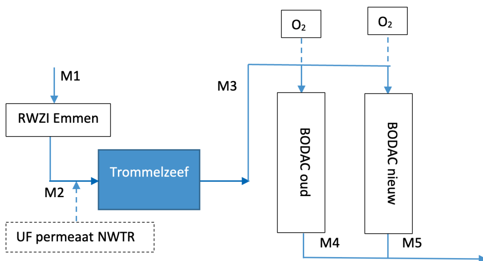
FIGUUR 2.1 VEREENVOUDIGD PFD VAN DE PROEFINSTALLATIE MET TWEE PARALLELLE BODAC FILTERS: OUD (RIJPE KOOL, NWTR FULL SCALE) EN NIEUW (VERSE KOOL). MONSTERPUNTEN M1 (RWZI INFLUENT), M2 (RWZI EFFLUENT), M3 (VOEDING BODAC), M4 (FILTRAAT BODAC OUD) EN M5 (FILTRAAT BODAC NIEUW)
