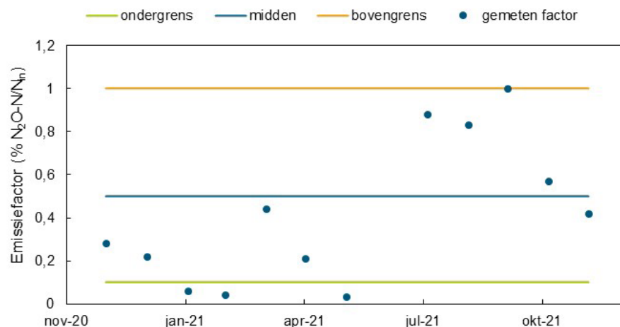
FIGUUR 2.2 GEMETEN EMISSIEFACTOR (MAANDWAARDEN) EN ONDER-MIDDEL-BOVEN GRENS VAN DE RISICOCATEGORIE GEMIDDELD VOOR HAAREN. ONDERGREN IS 0,1%, MIDDEN IS 0,5% EN BOVENGREN IS 1,0% (ZIE OOK TABEL 2.2)
