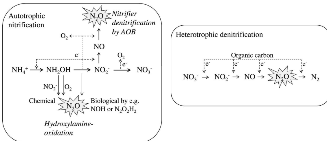
FIGUUR 4.1 OVERZICHT FORMATIEROUTES N_2O (WUNDERLIN ET AL. 2012)
