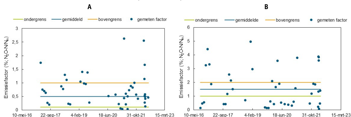
FIGUUR 2.8 GEMETEN EMISSIEFACTOR (MAANDWAARDEN) EN ONDER-MIDDEL- EN BOVENGRENS VOOR DE RISICOCATEGORIE LAAG (A) EN HOOG (B). VOOR DE RISICOCATEGORIE LAAG IS DE ONDERGRENS VOOR DE EMISSIEFACTOR 0,1%, IS DEZE 0,5% ALS GEMIDDELDE EN 1% IS DE BOVENGRENS. VOOR DE RISICOCATEGORIE HOOG IS DE ONDERGRENS VOOR DE EMISSIEFACTOR 1%, IS DEZE 1,5% ALS GEMIDDELDE EN 2% IS DE BOVENGRENS (ZIE OOK TABEL 2.4)
