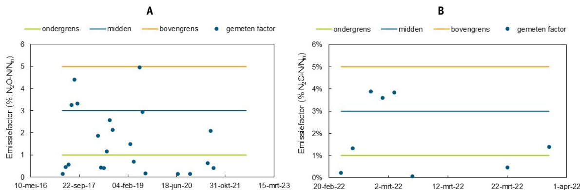
FIGUUR 2.3 GEMETEN EMISSIEFACTOR EN ONDER-MIDDEL-BOVEN GRENS VAN DE RISICOCATEGORIE HOOG VOOR A: AMSTERDAM WEST (MAANDWAARDEN) EN B: SCHIPHOL (DAGWAARDEN). ONDERGRENS IS 1%, MIDDEN IS 3% EN BOVENGRENS IS 5% (ZIE OOK TABEL 2.2)
