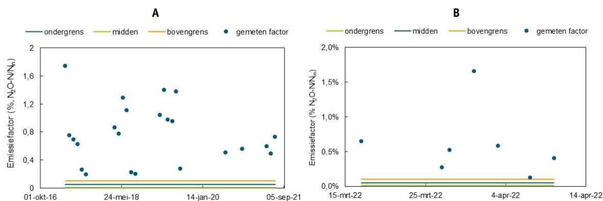
FIGUUR 2.1 GEMETEN EMISSIEFACTOR EN ONDER-MIDDEL-BOVEN GRENS VAN DE RISICOCATEGORIE LAAG VOOR A: AMSTERDAM WEST (MAANDWAARDEN) EN B: SCHIPHOL (DAGWAARDEN). ONDERGREN IS 0,01%, MIDDEN IS 0,05% EN BOVENGREN IS 0,1% (ZIE OOK TABEL 2.2)
