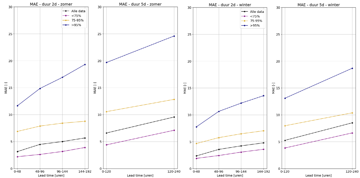
FIGUUR 13 GEMIDDELTE ABSOLUTE FOUT VOOR DE NEERSLAG UIT ECMWF EPS VOOR DE ZOMER (LINKER TWEE PANELEN) EN DE WINTER (RECHTER TWEE PANELEN). RESULTATEN VOOR DUREN VAN ZOWEL 2 ALS 5 DAGEN WORDEN GETOOND. DE RELATIEVE VERSCHILLEN VOOR DE RMSE ZIJN VRIJWEL IDENTIEK
