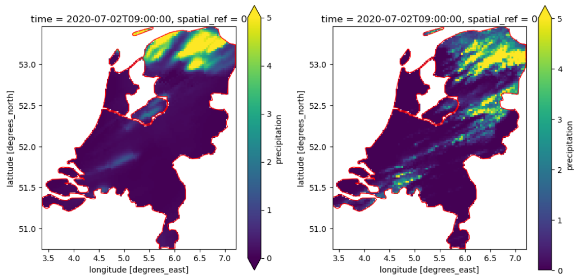
FIGUUR 14 ILLUSTRATIE VAN DE RASTERS ZOALS WE DIE GEBRUIKEN IN DE RUIMTELIJKE ANALYSE. LINKS HARMONIE40, RECHTS HET IRC. DE RODE LIJN GEEFT DE LANDSGRENS EN/OF KUSTLIJN WEE
