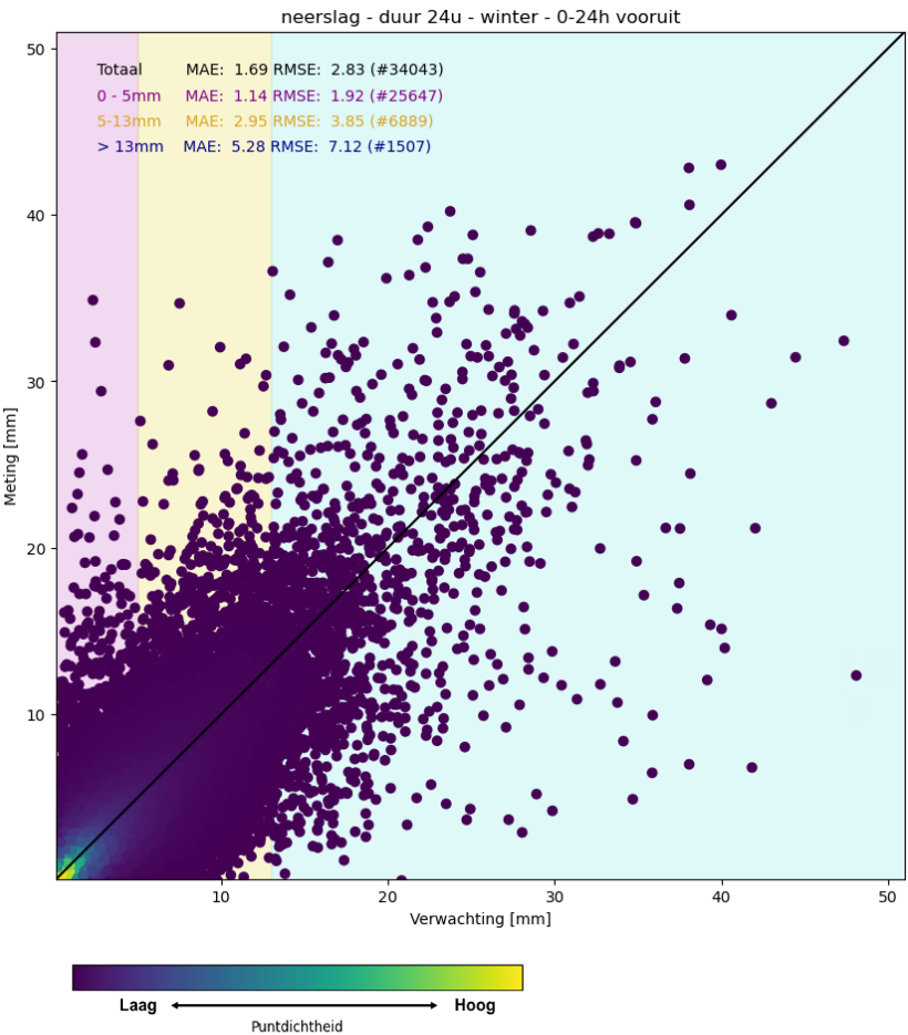
FIGUUR 2 VOORBEELDFIGUUR OM DE SCATTERPLOT TE ILLUSTREREN WAARMEE WE DE RESULTATEN BESCHRIJVEN. HET FIGUUR TOONT DE PUNTENWOLK MET DE PUNTDICHTHEID IN KLEUR. VOOR EEN AANTAL NEERSLAGKLASSEN (WEERGEGEVEN DOOR DE KLEURENVLAKKEN OP DE ACHTERGROND), WORDEN DE PRESTATIE-INDICES MAE EN RMSE BEREKEND
