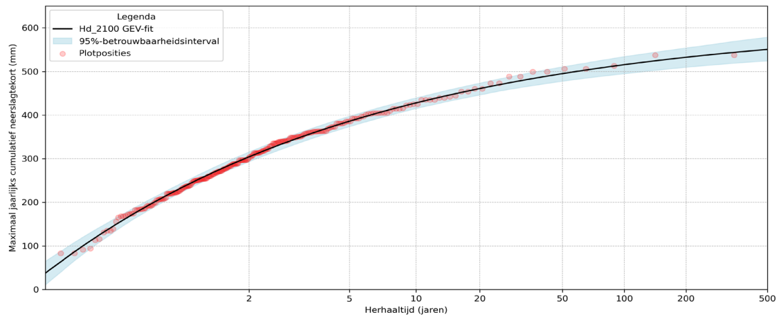
Figuur 28 Kansverdelingsfit voor Hd_2100
