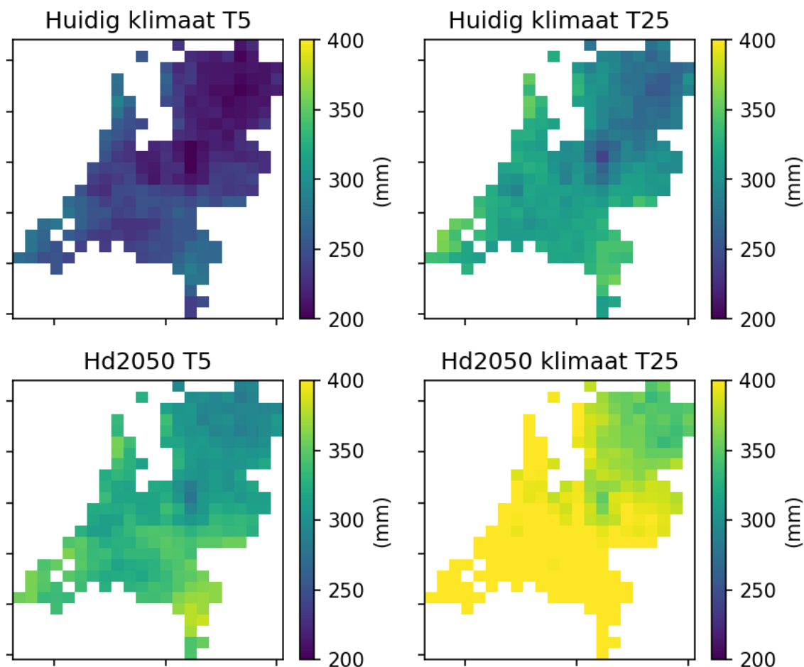
Figuur 11 Ruimtelijke variatie van het maximaal cumulatief neerslagtekort in het huidige klimaat en in het Hd2050-scenario bij herhalings tijden van vijf en vijfentwintig jaar. Het kleurverschil per paneel toont steeds een verschil van 200 mm
