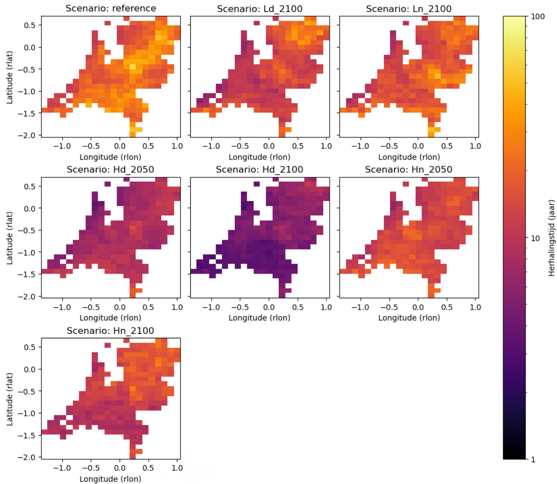
Figuur 15 Ruimtelijke variatie in herhalingsstijd per klimaatscenario bij een minimale 45-daagse neerslagsom van 12 mm
