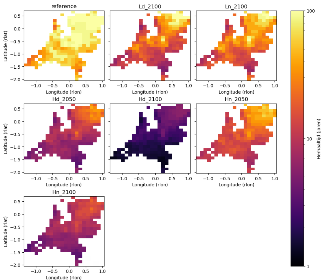
Figuur 13 Ruimtelijke variatie in herhalingstijd per klimaatscenario bij een maximaal cumulatief neerslagtekort van 350 mm
