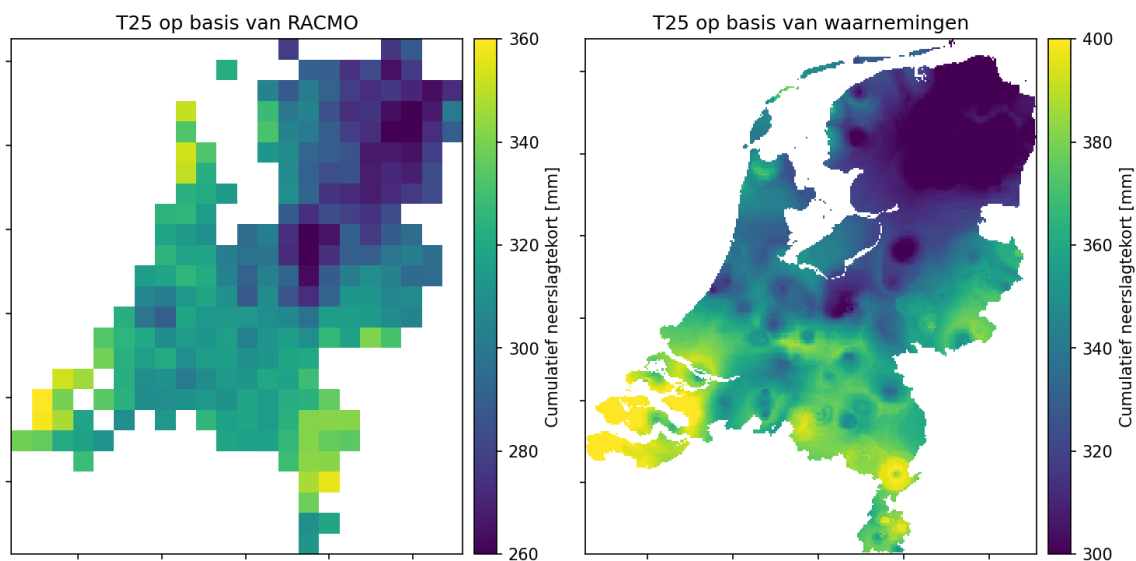
Figuur 12 Ruimtelijke variatie van het maximale cumulatieve neerslagtekort met een herhalingsjijd van 25 jaar voor de huidige situatie op basis van RACMO (links) en waarnemingen, afkomstig uit STOWA (2023) (rechts). Ter verduidelijking van de ruimtelijke verschillen wijken de kleurschalen van beide panelen licht af
