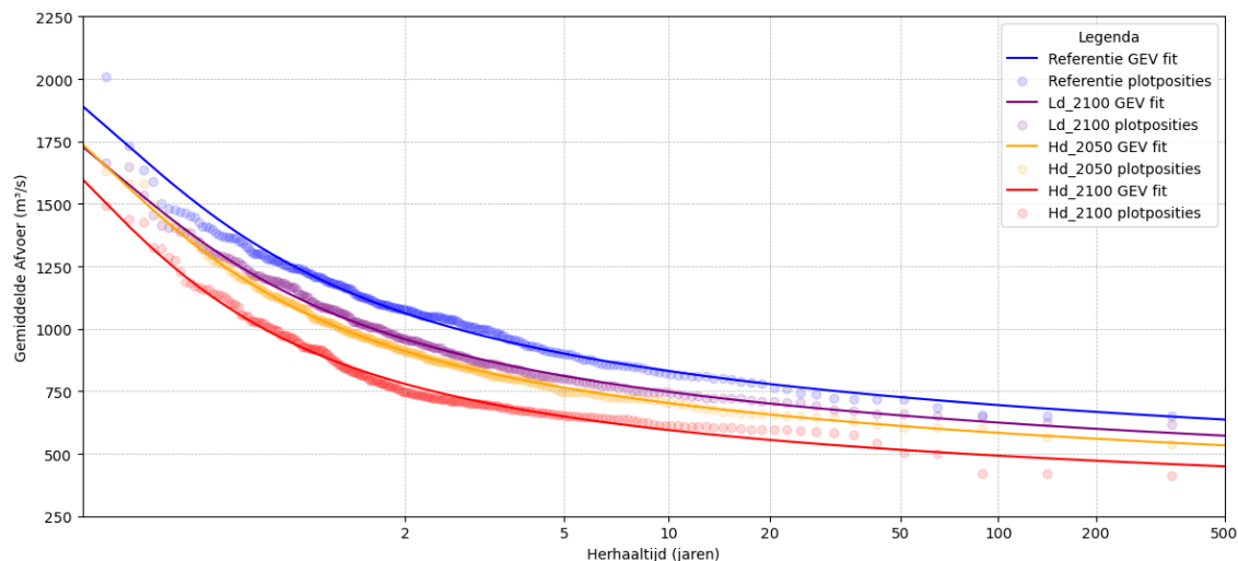
Figuur 7 Minimale zevendaagse Rijnafoer als functie van de geschatte herhalingstijd voor de onderzochte KNMI'23-scenario's
