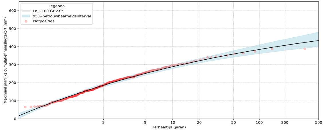
Figuur 30 Kansverdelingsfit voor Ln2100
