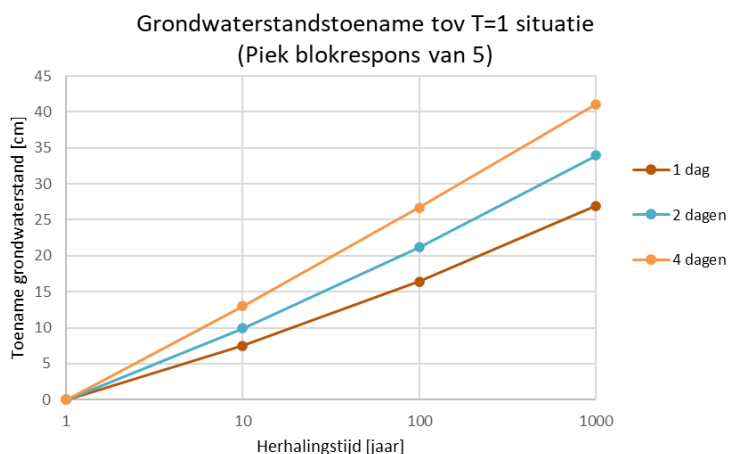
Figuur 22 De grondwaterstandstoename ten opzichte van de T=1 jaar-situatie voor verschillende neerslagduren
