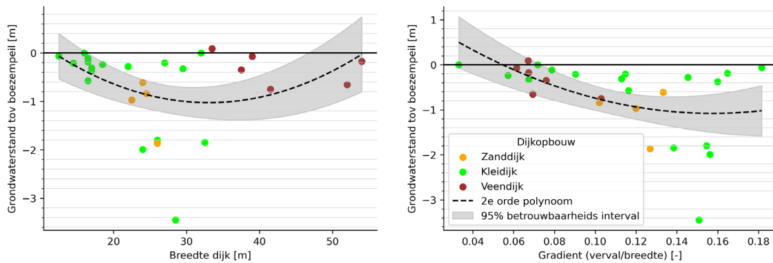
Figuur 17 De grondwaterstand bij de binnenkruin ten opzichte van het boezempeil uitgezet tegenover geometrische kenmerken van de dijk, namelijk de breedte (links) en de gradiënt (rechts)
