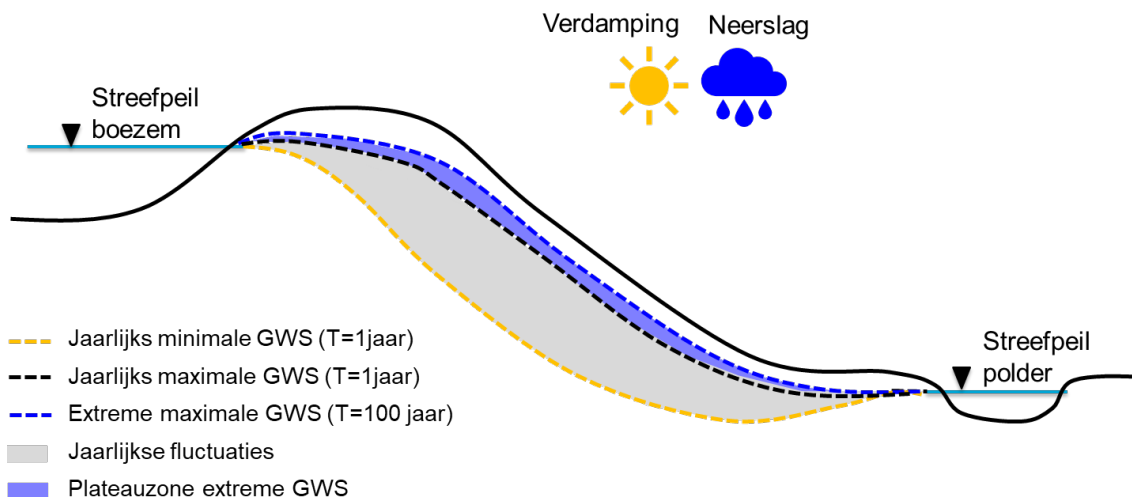
Figuur 19 Schematische weergave van de variatie van de freatische lijn binnen het jaar (grijze vlak) en de plateauzone waarbinnen de freatische lijn fluctueert bij extreme situaties (blauwe vlak)
