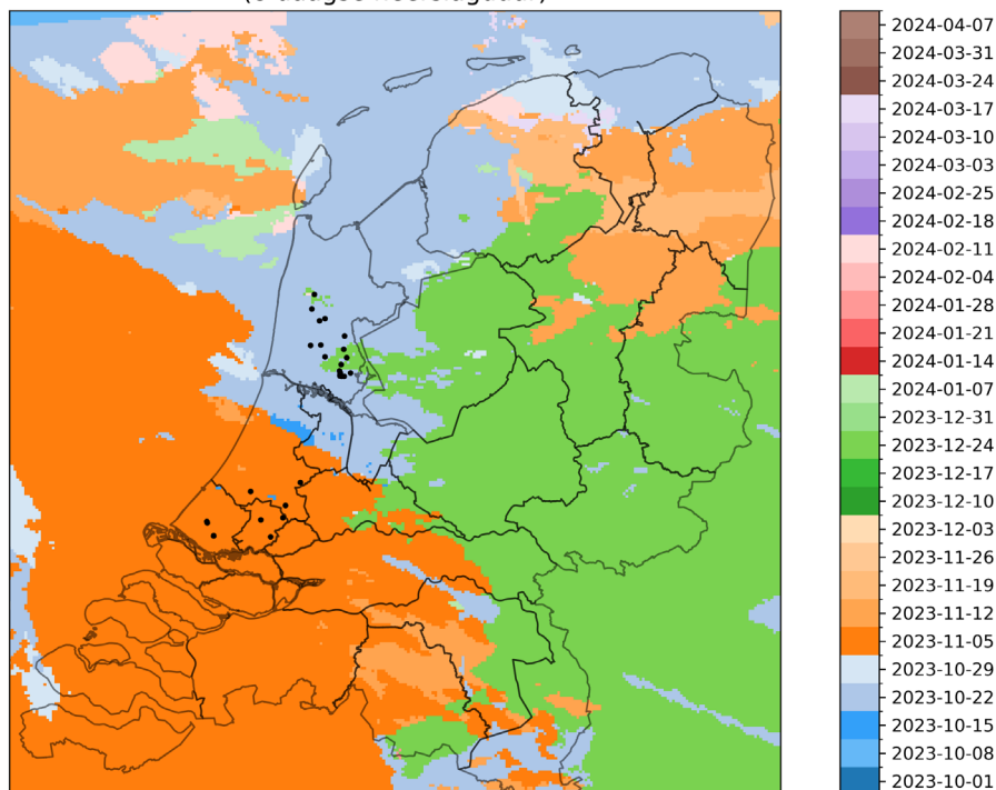
Periode maximale neerslaghoeveelheid (8 daagse neerslagduur)
