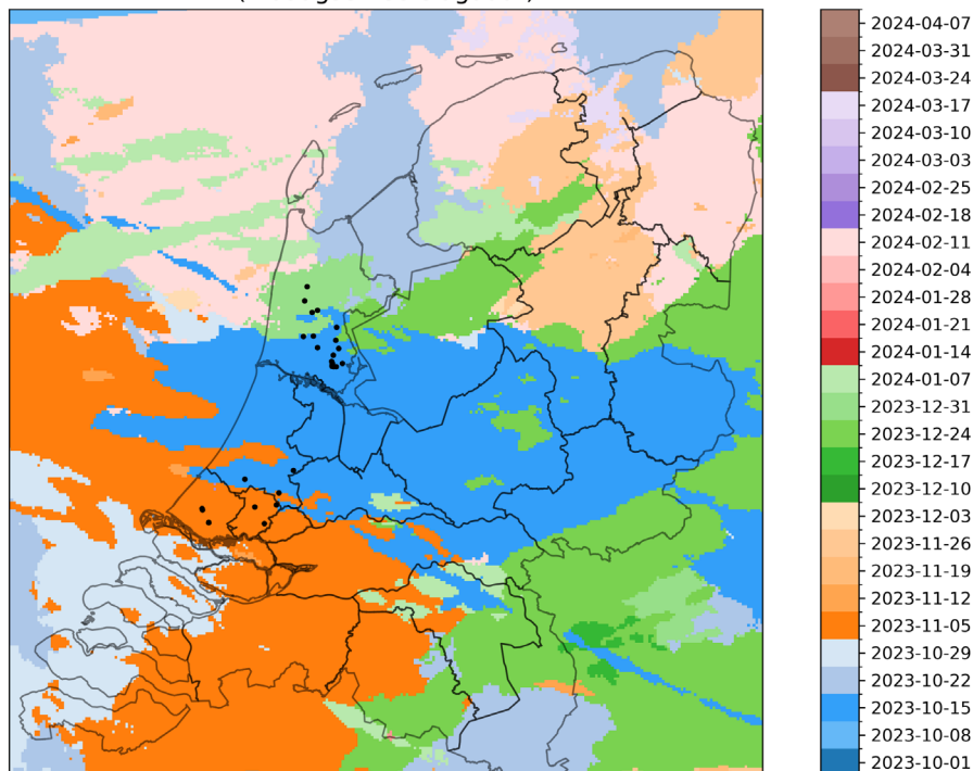
Periode maximale neerslaghoeveelheid (4 daagse neerslagduur)
