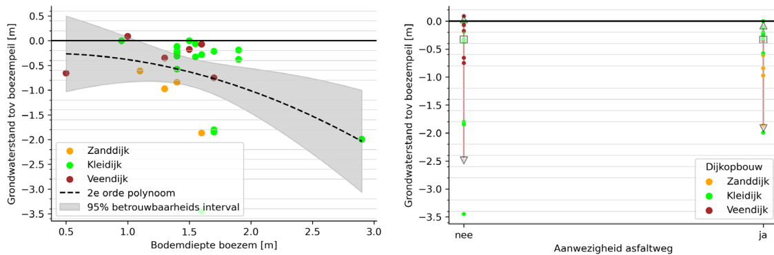
Figuur 18 De grondwaterstand bij de binnenkruin ten opzichte van het boezempeil uitgezet tegenover de bodemdiepte van de boezem (links) en de aanwezigheid van een asfaltweg op de kruin (rechts)
