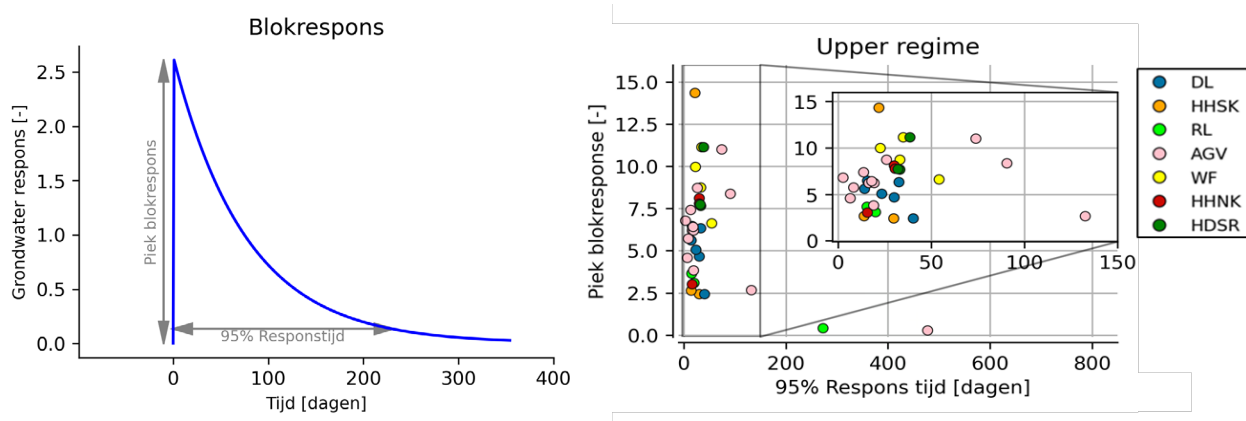
Figuur 21 Links: visualisatie van de piekblokrespons en de 95% responstijd van de impulsresponsefunctie. Rechts: de karakteristieke kenmerken van de tijdreeksmodellen opgesteld voor 35 peilbuizen in het talud van verschillende boezem- en polderkaden, waarbij de kleuren aangeven binnen welk waterschap de kade ligt (uit Strijker & Kok (2024))
