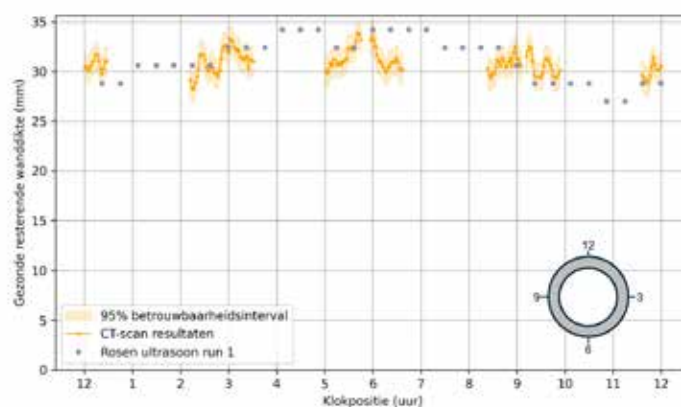
Figuur 4.23 Inspectieresultaten van Rosenxt voor de gezonde resterende wanddikte van buisdeel 139 op een afstand van 603,25 m vanaf het rioolgemaal, tezamen met de CT-scan resultaten
