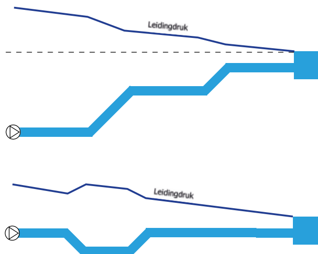
Figuur 4.9 Schematische weergave van de persleidingdruk in een hellend (boven) en vlak (onder) gebied
