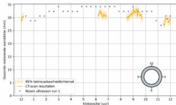
Figuur 4.22 Inspectieresultaten van Rosenxt voor de gezonde resterende wanddikte van buisdeel 137 op een afstand van 594,11 m vanaf het rioolgemaal, tezamen met de CT-scan resultaten
