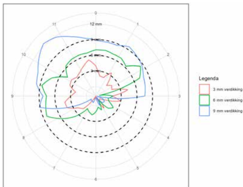
Figuur 4.21 Dikte van de aangesmeerde delen per klokpositie, berekend door uit de inline-inspectieresultaten het verschil in gezonde resterende wanddikte voor en op het verdikte gedeelte te nemen.
