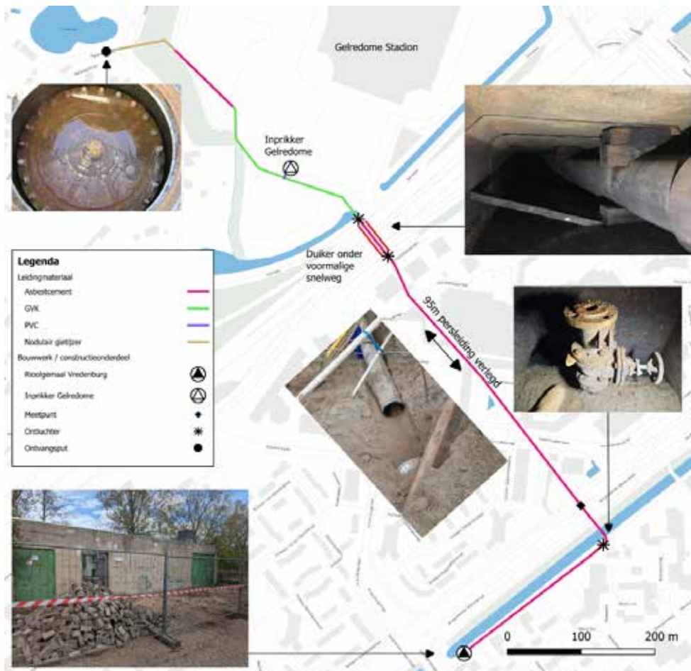
Figuur 2.1 Tracéverloop persleiding Vredenburg. Het tracé begint bij rioolgemeal Vredenburg in het zuiden en eindigt bij de uitstroompuit in het noorden.
