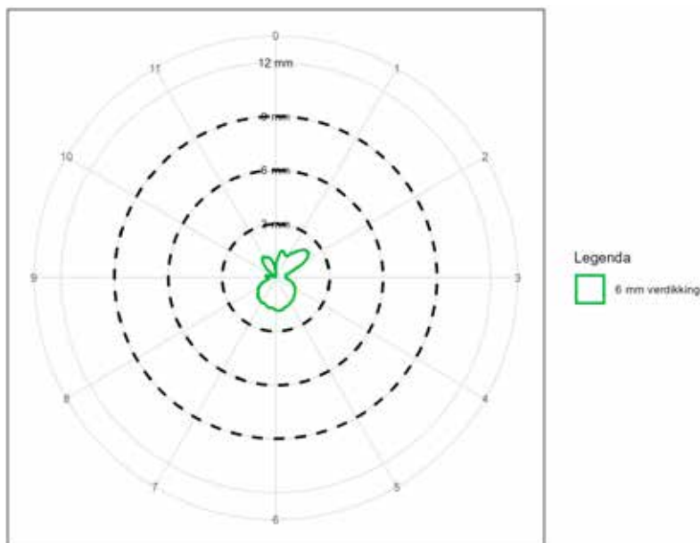
Figuur 4.26 Dikte van de aangesmeerde delen per klokpositie, berekend door uit de inline-inspectieresultaten het verschil in uitgeloopte wanddikte voor en op het verdikte gedeelte te nemen.
