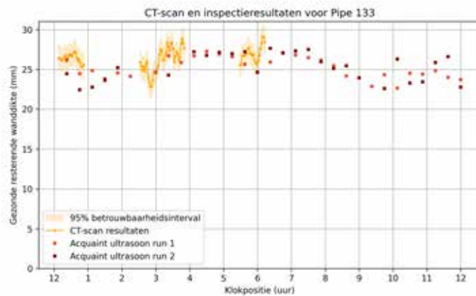
Figuur 4.16 Inspectieresultaten van Acquaint voor de gezonde resterende wanddikte van buisdeel 133 op een afstand van 581,81m vanaf het gemaal, tezamen met de CT-scan resultaten
