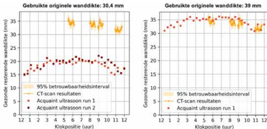
Figuur 4.18 Effect van de gebruikte originele wanddikte op de resultaten voor de gezonde resterende wanddikte voor buisdeel 137 op 597,64 m. Links is een originele wanddikte van 30,4 mm gebruikt en rechts een wanddikte van 39 mm, wat de wanddikte is die ook uit de CT-scan resultaten volgde.
