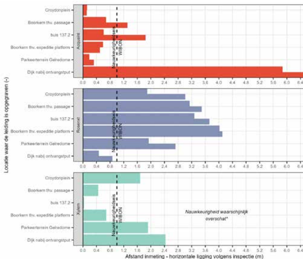
Figuur 4.4 Verschil tussen de ingemeten leidingligging en de inspectieresultaten. *Xylem heeft alleen één samengevoegd resultaat gerapporteerd, wat mogelijk leidt tot een overoptimistische nauwkeurigheid.
