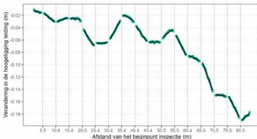
Figuur 4.28 Hoogteligging van de gemeten buisdelen ten opzichte van het beginpunt
