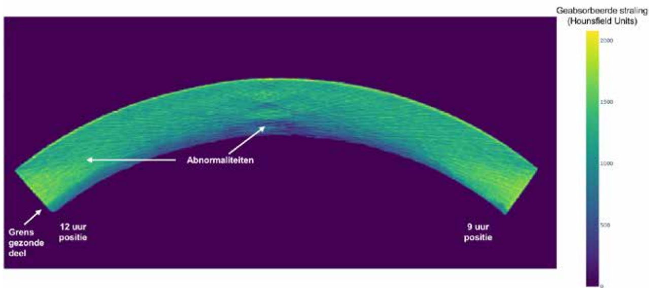
Figuur 4.12 Voorbeeld van een CT-scan doorsnede met links de bovenkant van de buis (12 uur positie). De donkere delen met een lagere stralingsdichtheid zijn uitgelooft.
